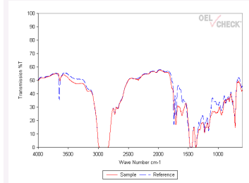
红外光谱
